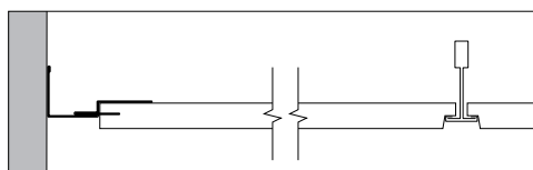
5. Vinkelkantprofil med kantclips
